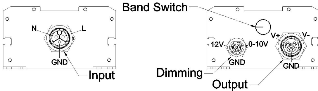
-CJJ3/-CLL3 End Cap
