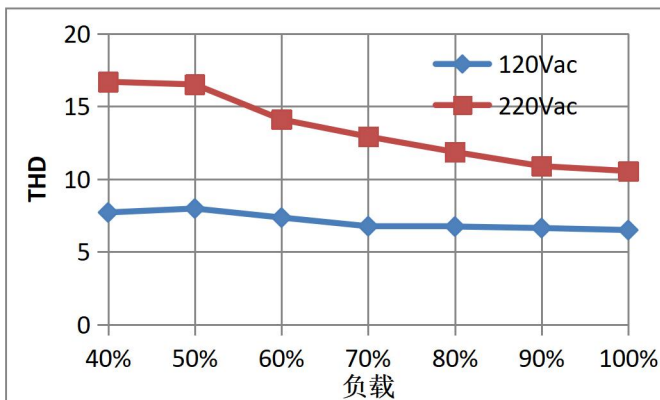
THD - 负载曲线
