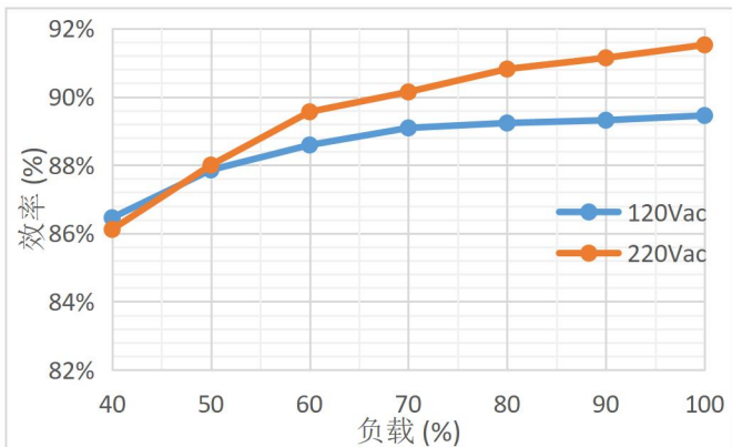
效率-负载曲线
